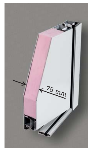
Oboustranně překrytá výplň, tloušťka 75 mm. U_d = \text{od } 1,0 \text{ W/m}^2\text{K}
