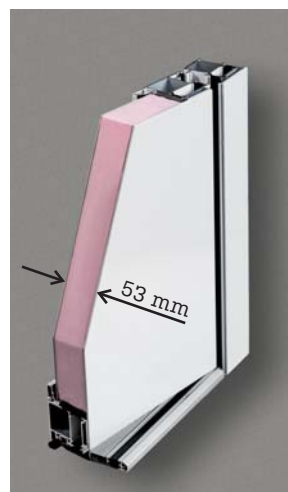
Jednostranně překrytá výplň, tloušťka 53 mm. U_d = \text{od } 1,2 \text{ W/m}^2\text{K}
