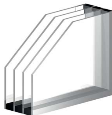
čtyřsklo 4-18-4-18-4-18-4 (čiré-matelux-matelux-čiré)
